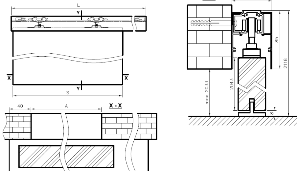
Rys. 2. Montaż systemu Spazio CD
