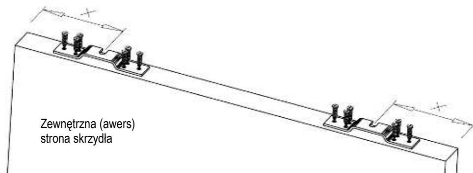
Rys. 3. Montaż uchwytów do skrzydła przesuwnego.
