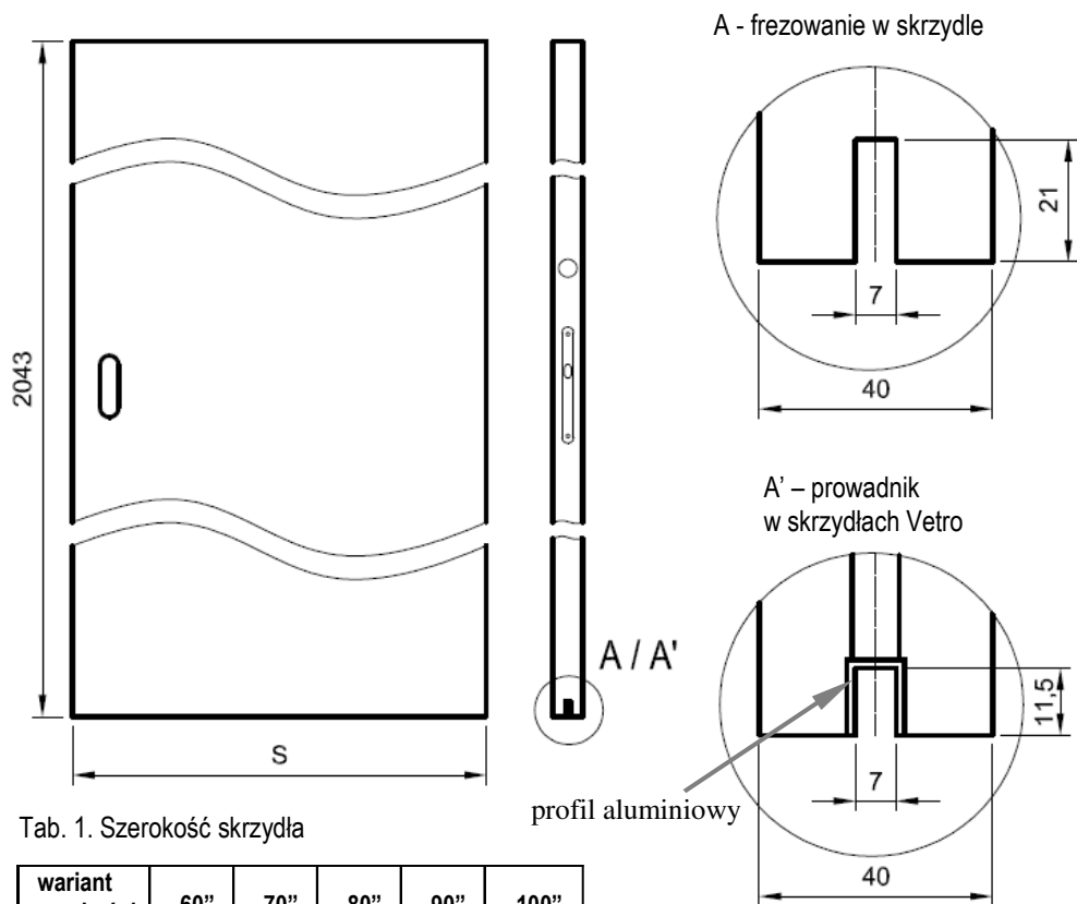
Rys. 1. Skrzydło drzwiowe przesuwne
